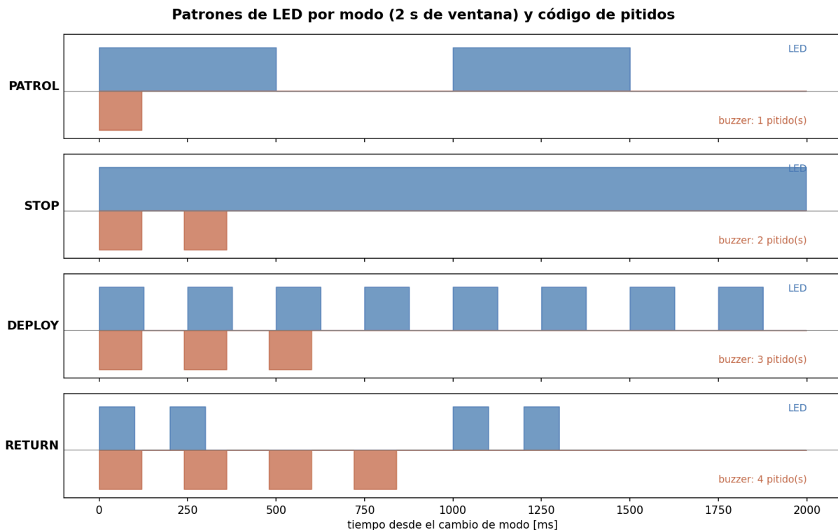
Patrones de LED por modo y código de pitidos del buzzer en el cambio de modo.
