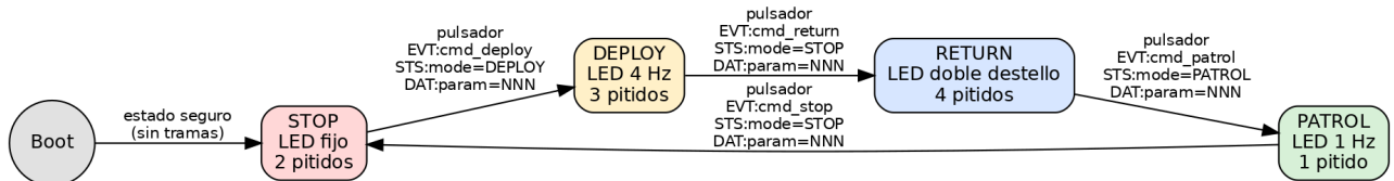
Diagrama de estados de la caja de comandos con las tramas emitidas en cada transición.
