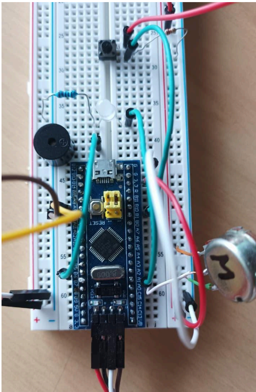
Montaje físico de la caja de comandos:
